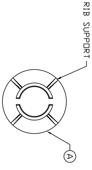
LID PLAN
